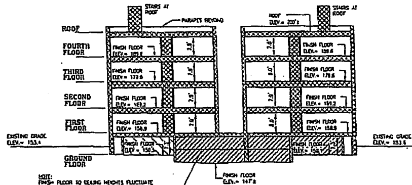
SECTION D-D
